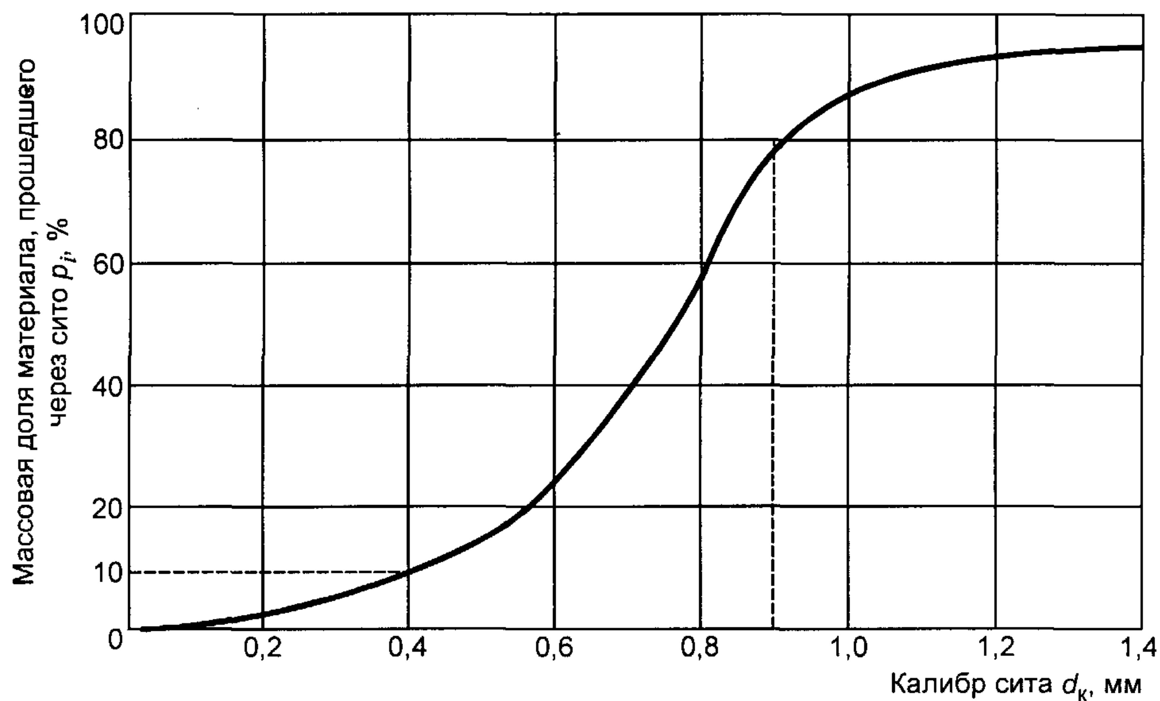
Рисунок А.1 — График ситового анализа материала
