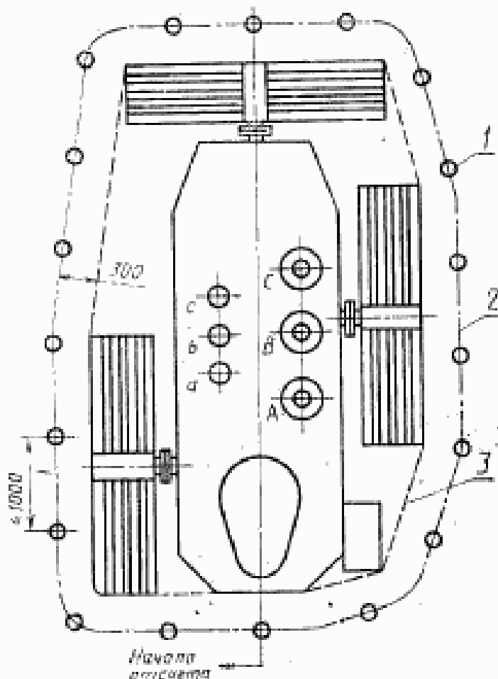
1 — микрофон; 2 — измерительная линия; 3 — излучающая поверхность
