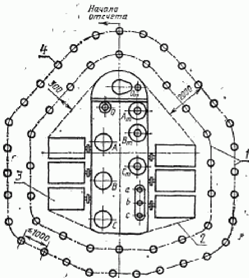
1 — измерительная линия; 2 — излучающая поверхность; 3 — охладитель; 4 — микрофон
