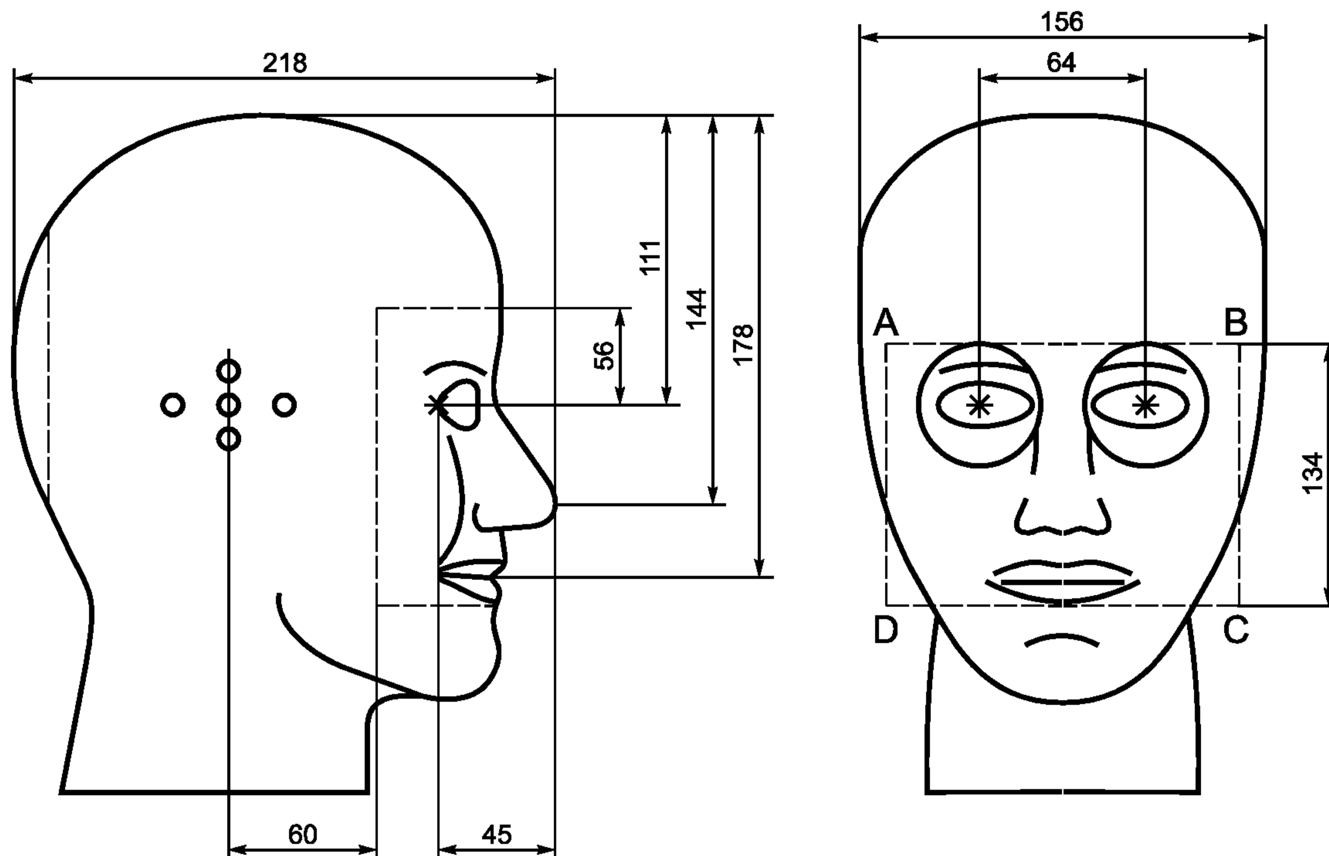
Рисунок 2 — Контрольный макет головы
