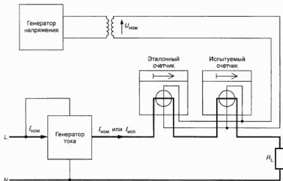
Рисунок А.1 — Схема испытательной цепи (справочная)
