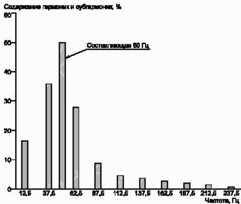
Рисунок А.3 — Распределение гармоник (анализ Фурье не завершен)
