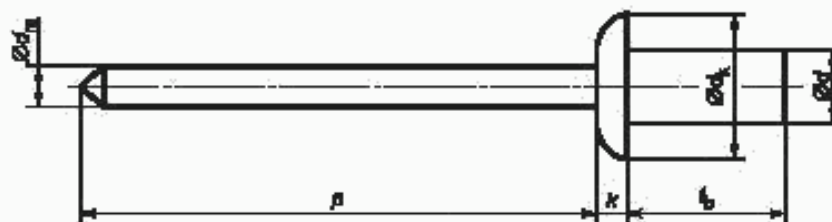
Рисунок 1 — Размеры заклепок
