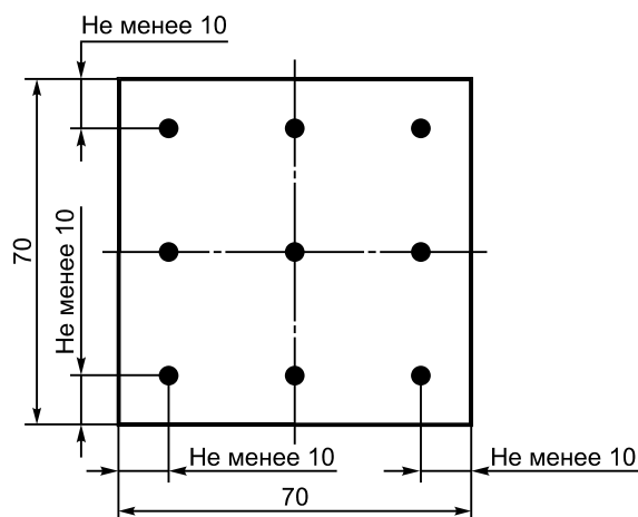
Рисунок 1 — Точки измерения толщины образца
