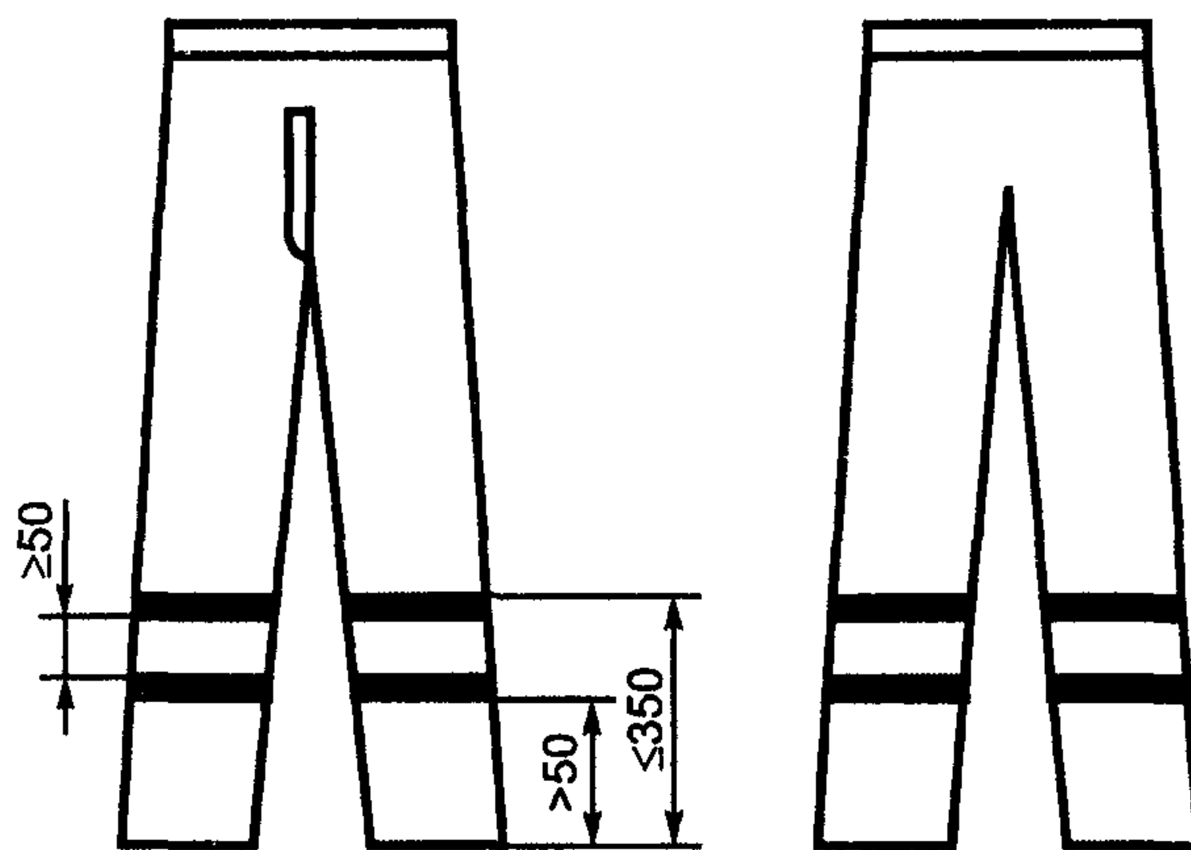
Рисунок Б.9 — Брюки
