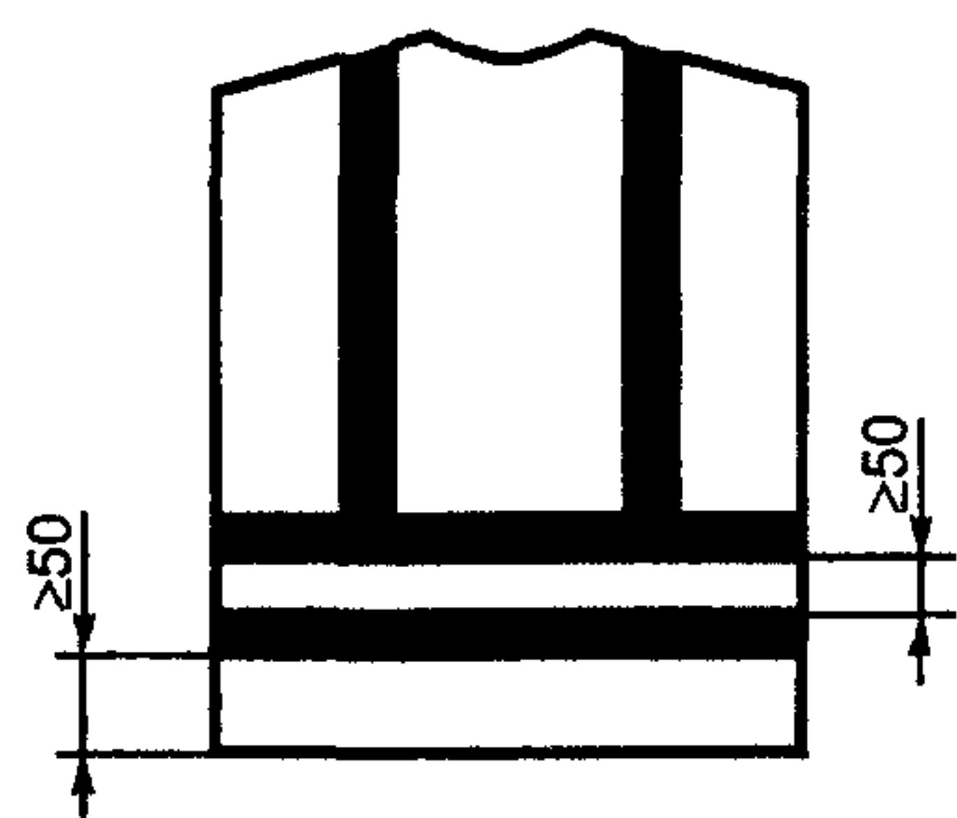
Рисунок Б.5 — Жилет-накидка
