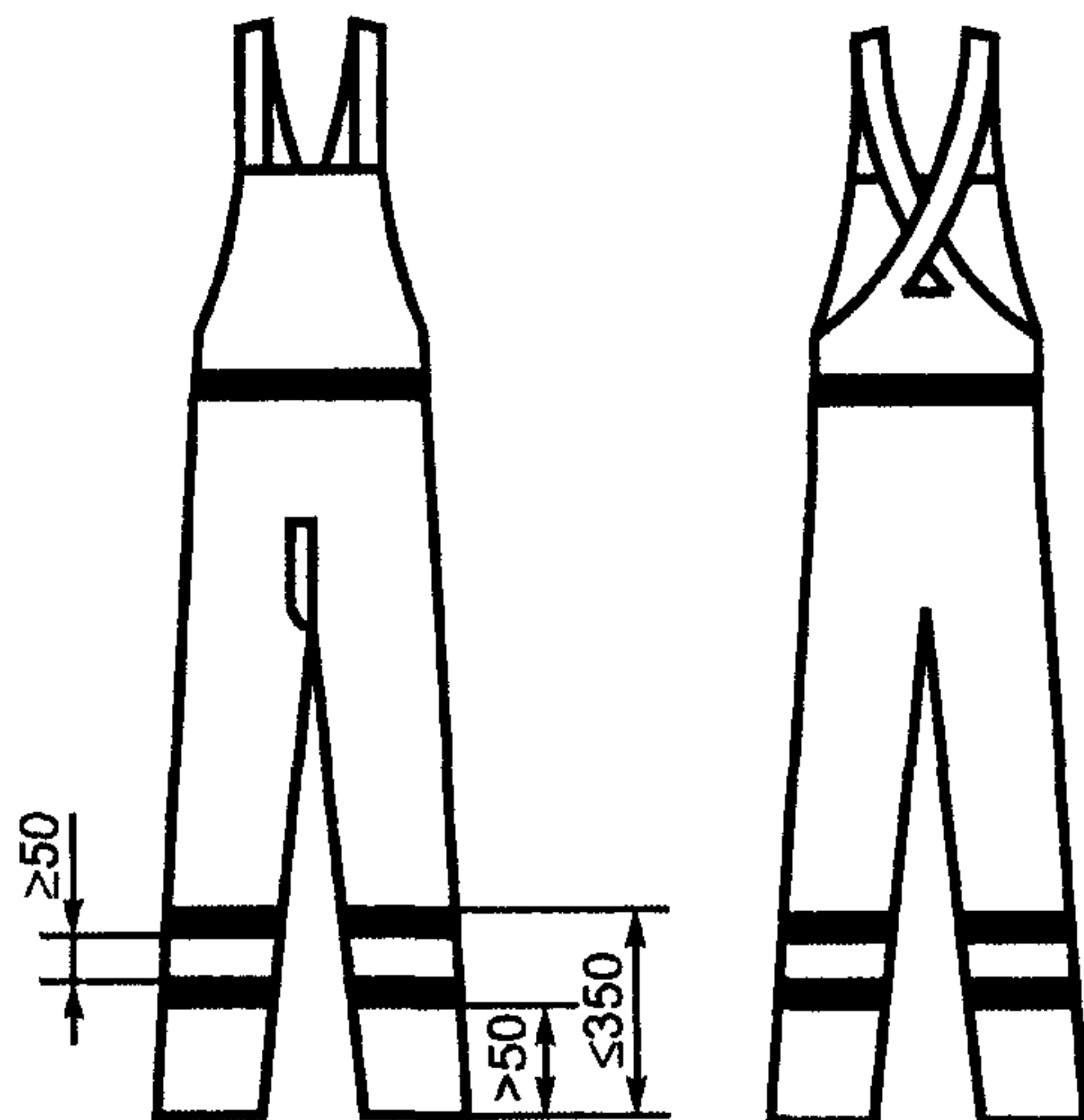
Рисунок Б.8 — Полукомбинезон
