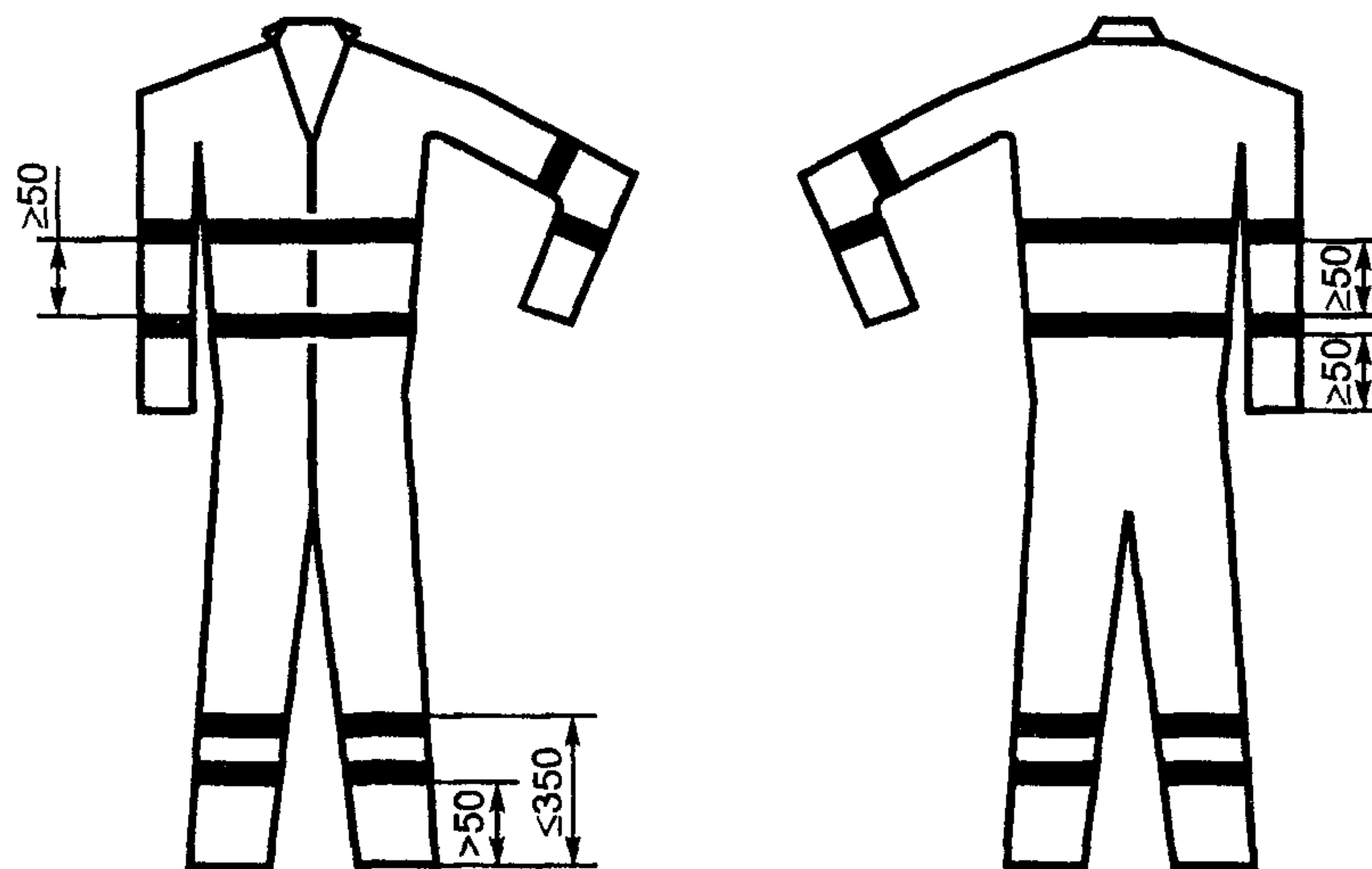
Рисунок Б.1 — Закрытый комбинезон
