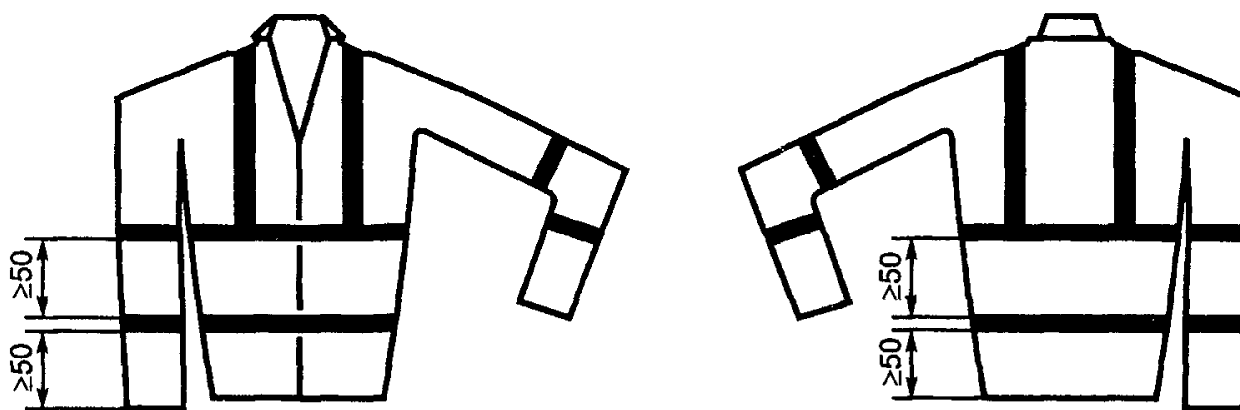
Рисунок Б.2 — Куртка
