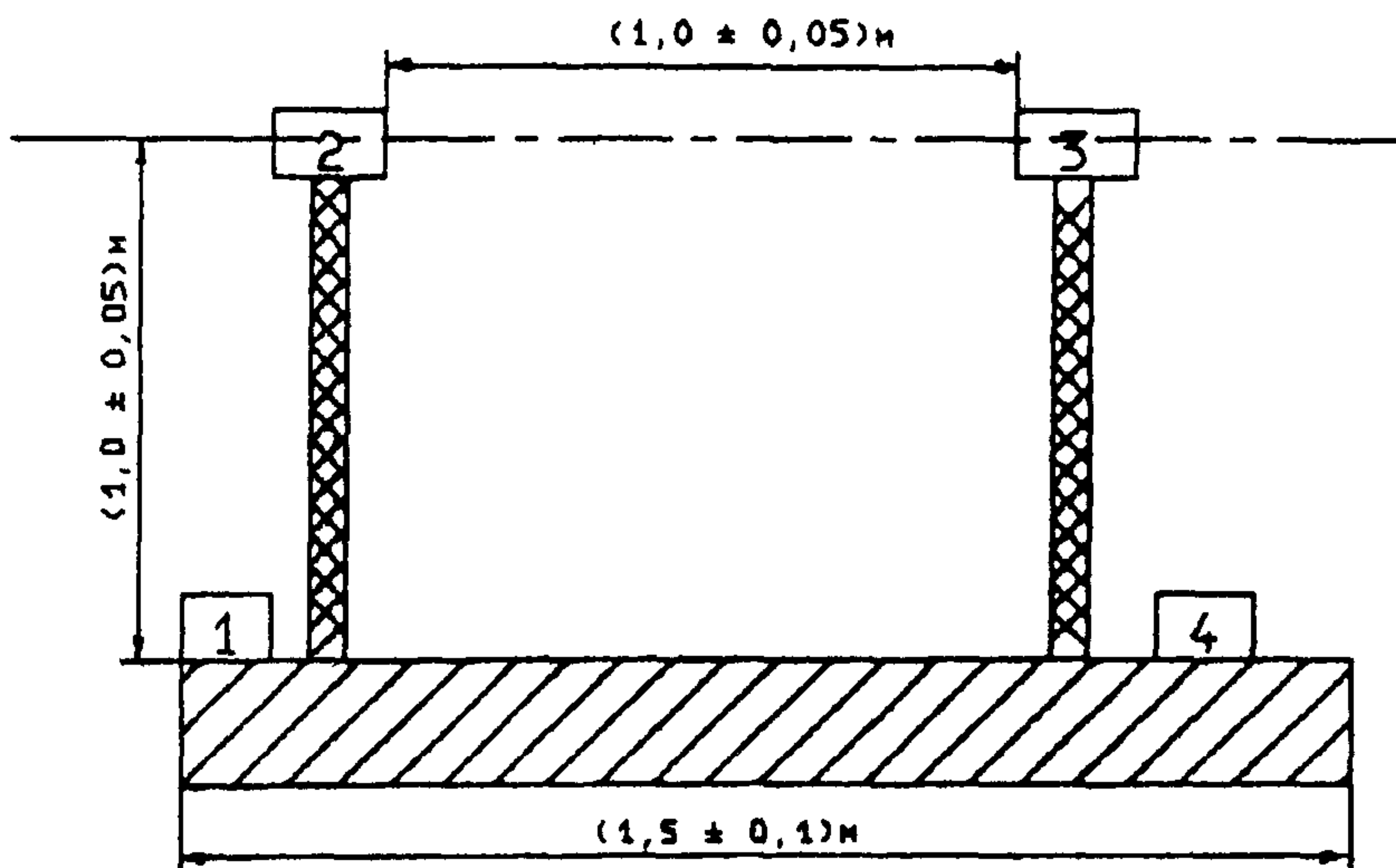
Стенд для проведения испытаний по измерению звукового давления:
