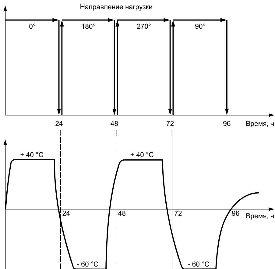
Рисунок 4 — Термомеханические испытания
