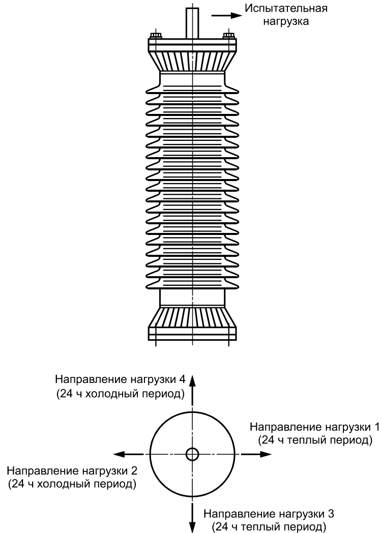
Рисунок 5 — Направления действия изгибающей нагрузки при термомеханических испытаниях
