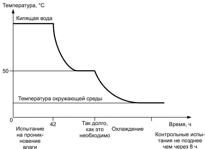
Рисунок 6 — Испытания на проникновение влаги
