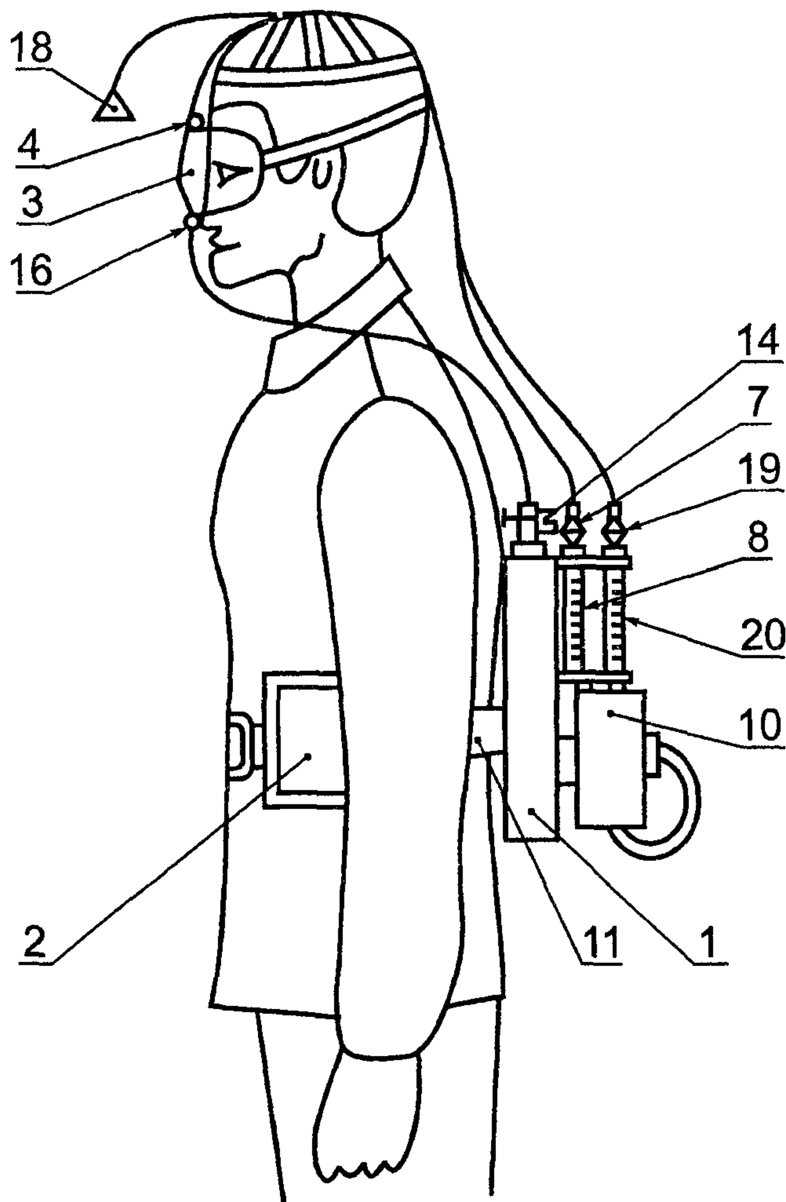
1 — автономный побудитель расхода воздуха, 2 — аккумулятор, 3 — очки, 4, 16 — заборный штуцер, 7, 19 — поглотители, 8, 20 — ротаметры, 10 — очиститель воздуха; 11 — крепежный гарнитур, 14 — регулировочный вентиль; 18 — пробоотборник
