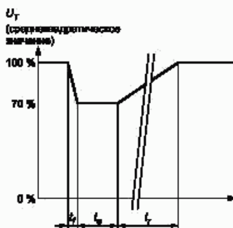
Рисунок 3 — Изменение напряжения
