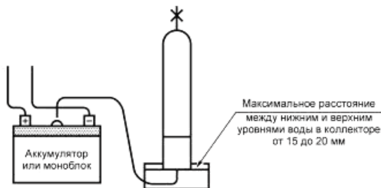
Рисунок 1 — Пример приспособления для сбора газа
