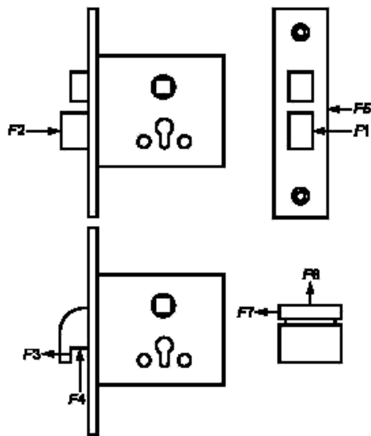
Рисунок 1 — Точки приложения сил, воздействующих на механизм замка
